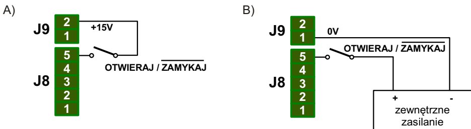
Rys. 3.6. Podłączenie sygnałów sterujących przy wykorzystaniu wejścia {OTWIERAJ} .
